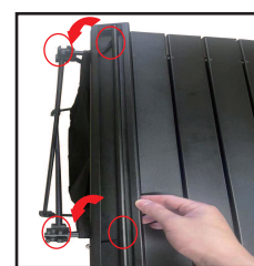
⑤天板を開き、天板裏面のパーツを両側のポールに押し込みます。
